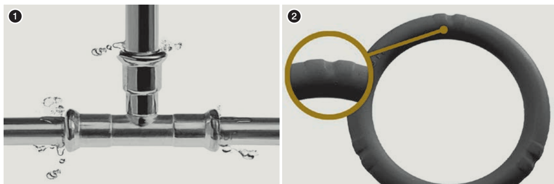
O-Ring LBP с функцией обнаружения неопрессованных соединений
