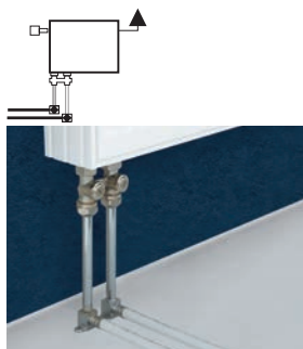
с присоединительными прямыми вентилем
