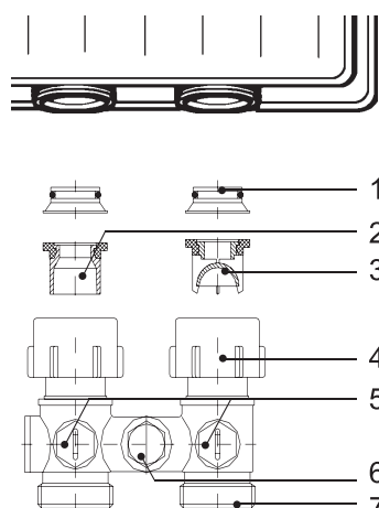
Узел подключения радиаторов с HP 3/4", D2 и E2
