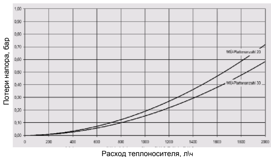
Диаграмма потери расхода в первичном контуре
