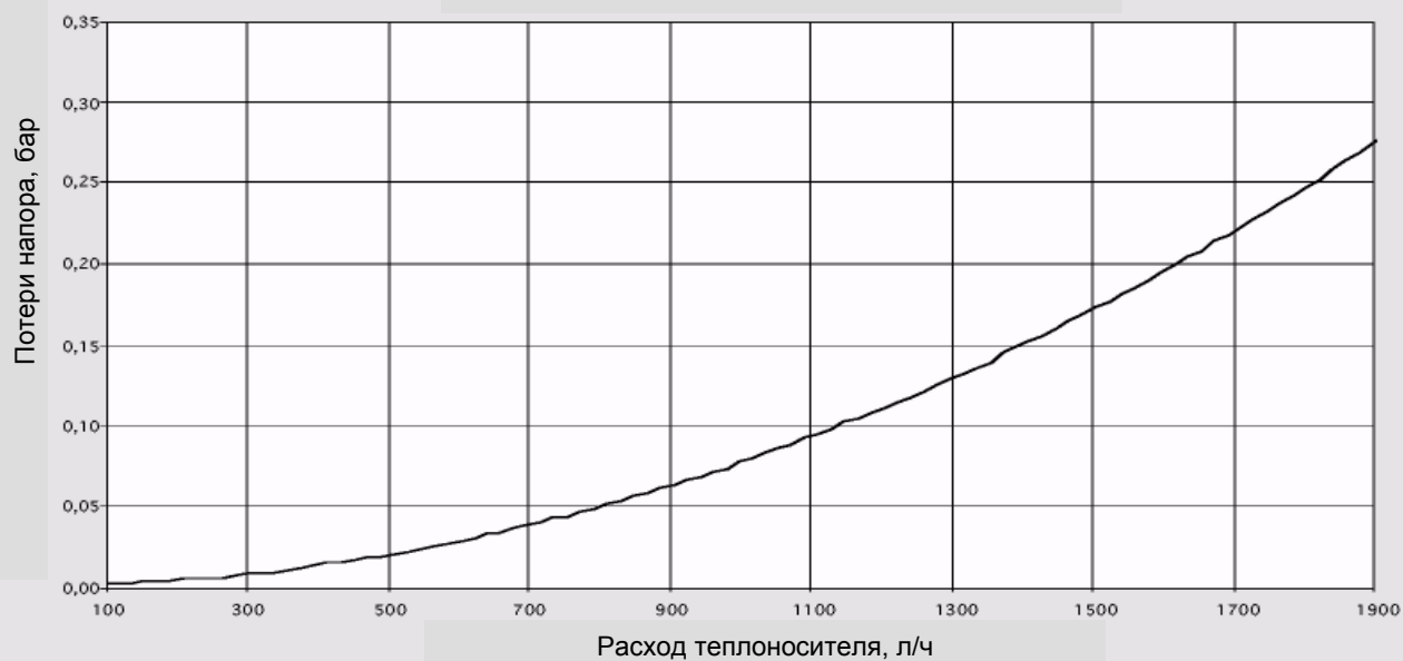
Диаграмма потери напора
