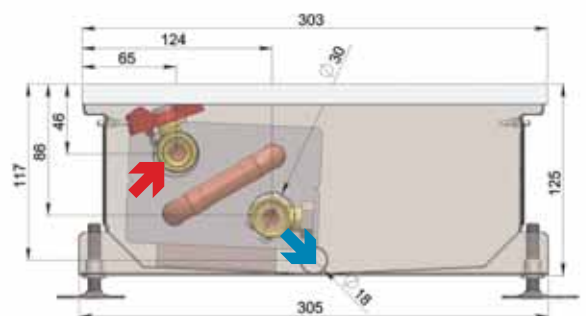
поперечный разрез
