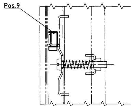
Einzelheit M2:1
