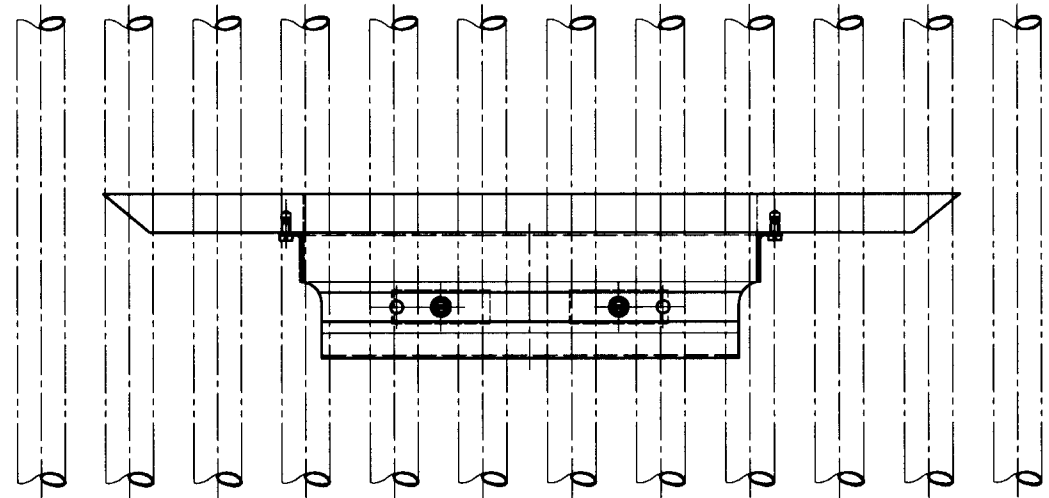
Einzelheit M2:1
