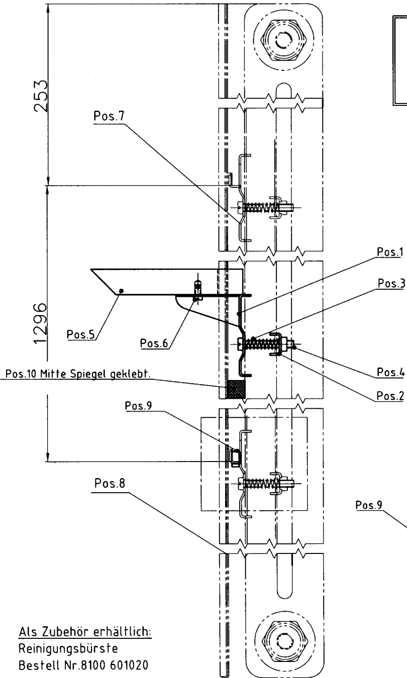
Einzelheit M2:1
